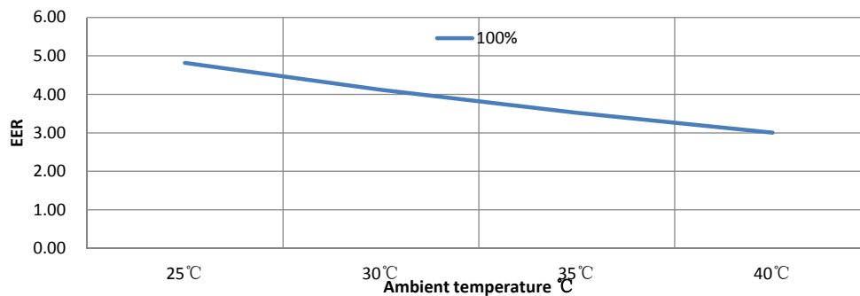
IXCR36 EER Curve
