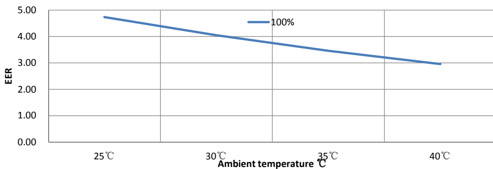
IXCR46 EER Curve
